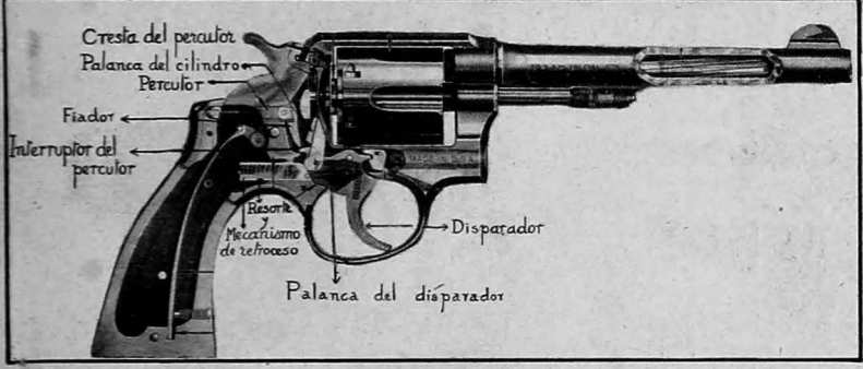
Corte transversal de un arma moderna, mostrando los mecanismos de seguridad que impiden el disparo del arma cuando no se ha oprimido el gatillo.
