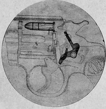
El seguro positivo de un revólver moderno. Las partes sombreadas constituyen el mecanismo que impide la percusión cuando no se ha oprimido el gatillo.
